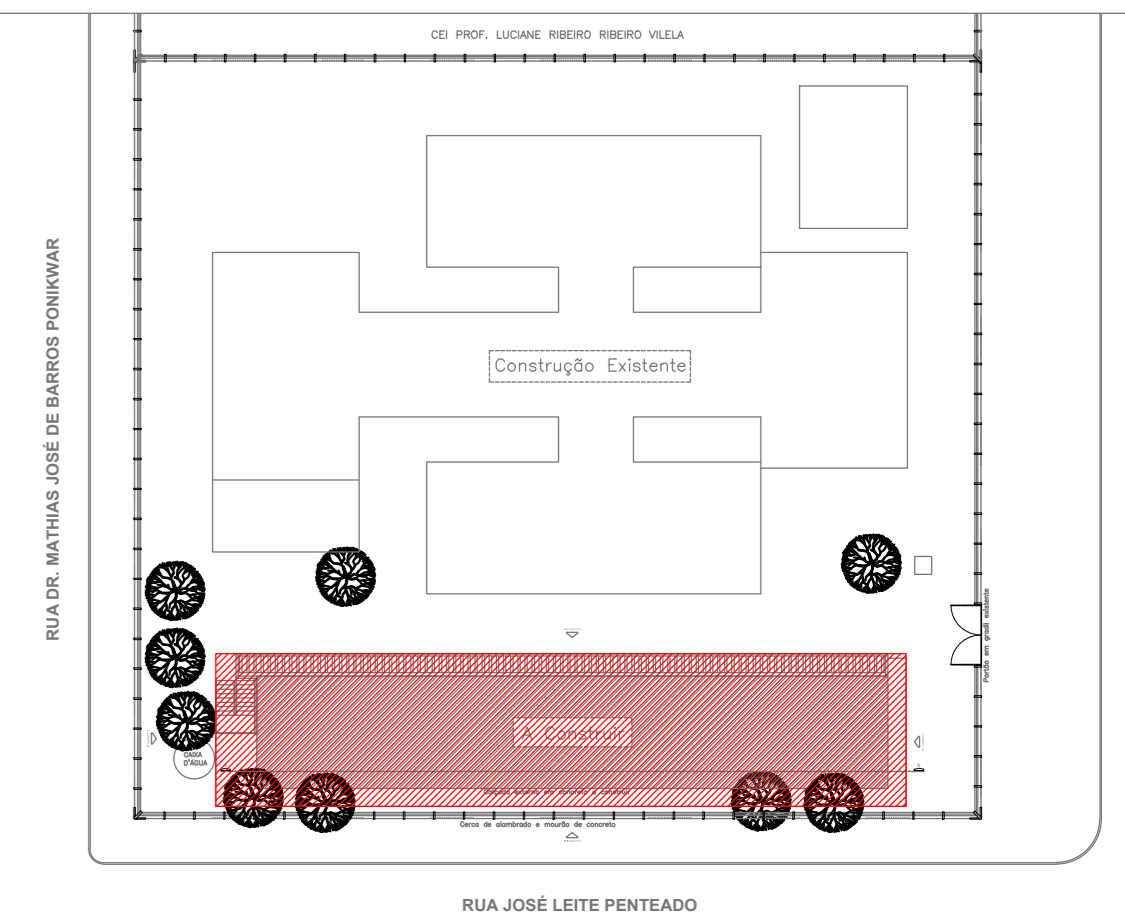
PLANTA DE LOCALIZAÇÃO - PRÉDIO ANEXO CASI ESCALA: 1:500
