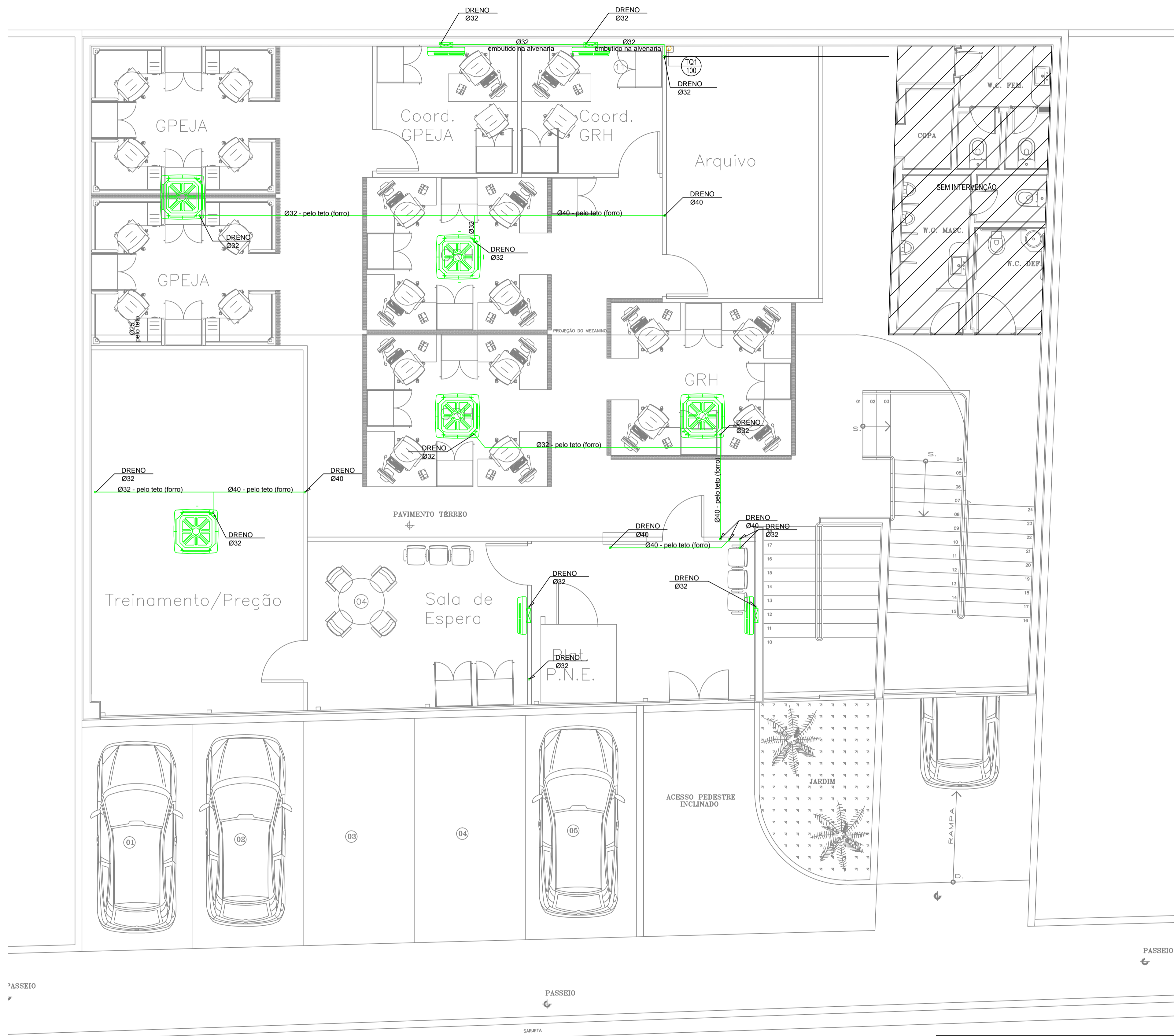
PLANTA DE DISTRIBUIÇÃO HIDRÁULICA - TÉRREO ESCALA: 1:50
