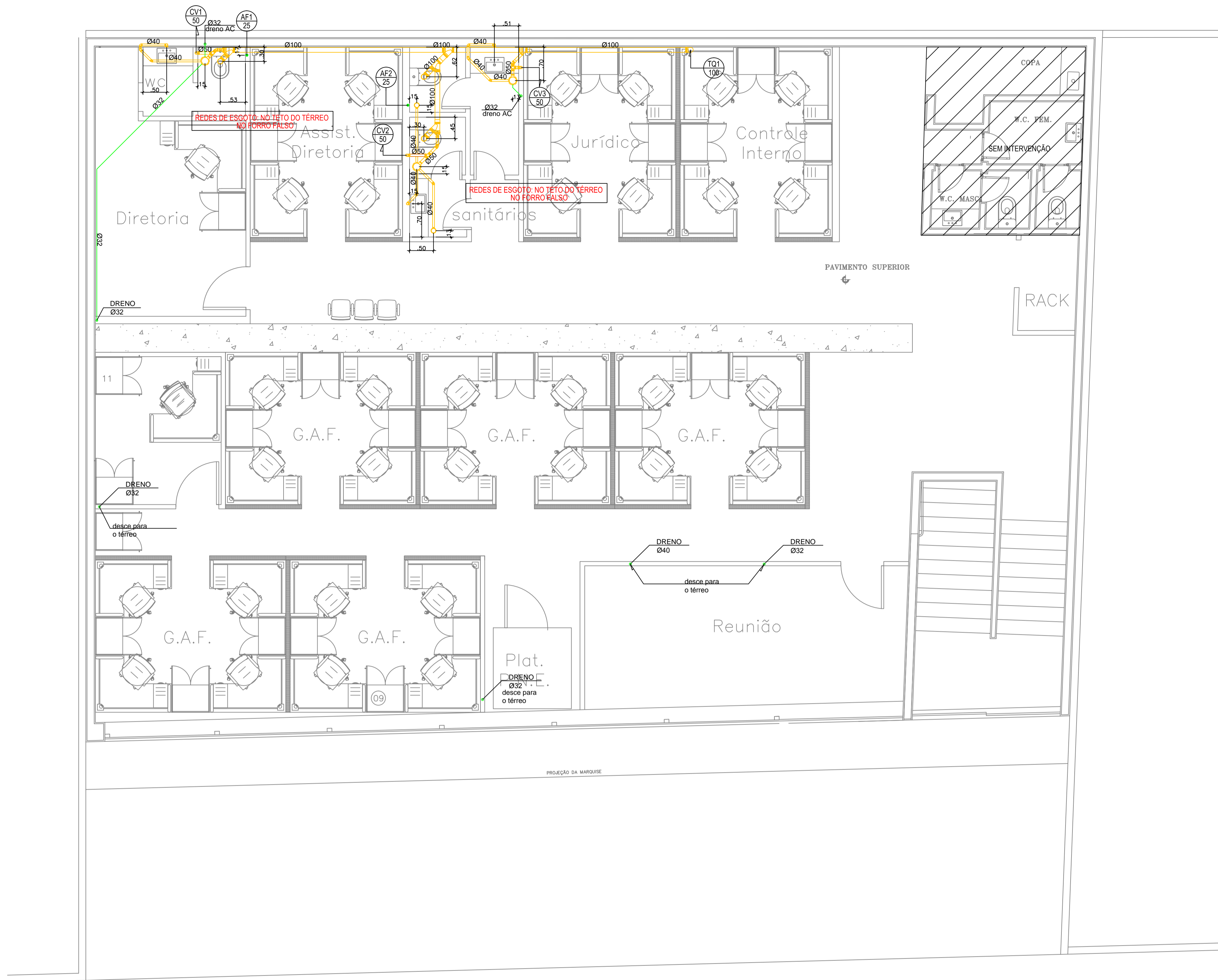
PLANTA DE DISTRIBUIÇÃO HIDRÁULICA - PISO MEZANINO ESCALA: 1:50
