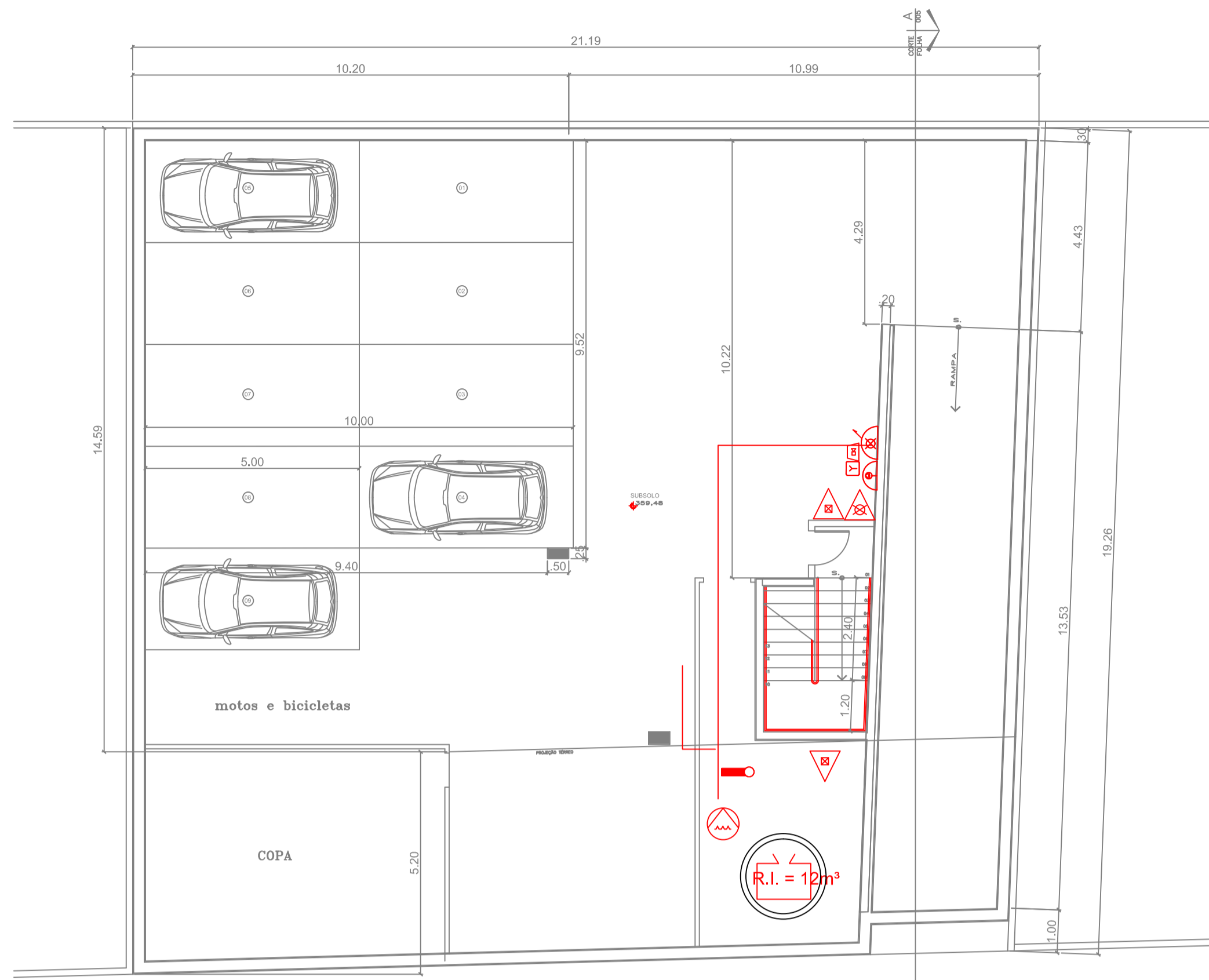
PLANTA BAIXA - SUBSOLO Escala 1:100
