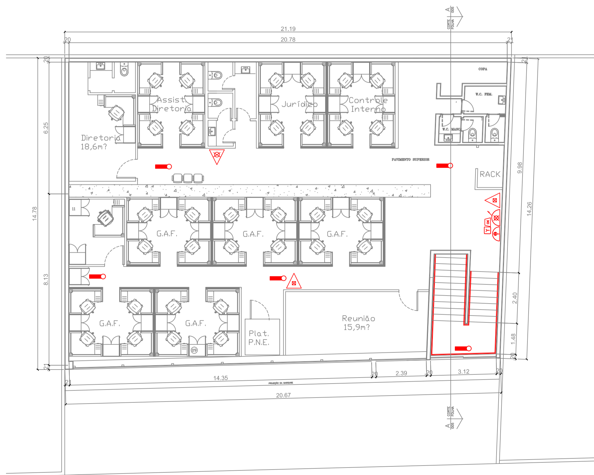
PLANTA BAIXA - PAVIMENTO MEZANINO Escala 1:100
