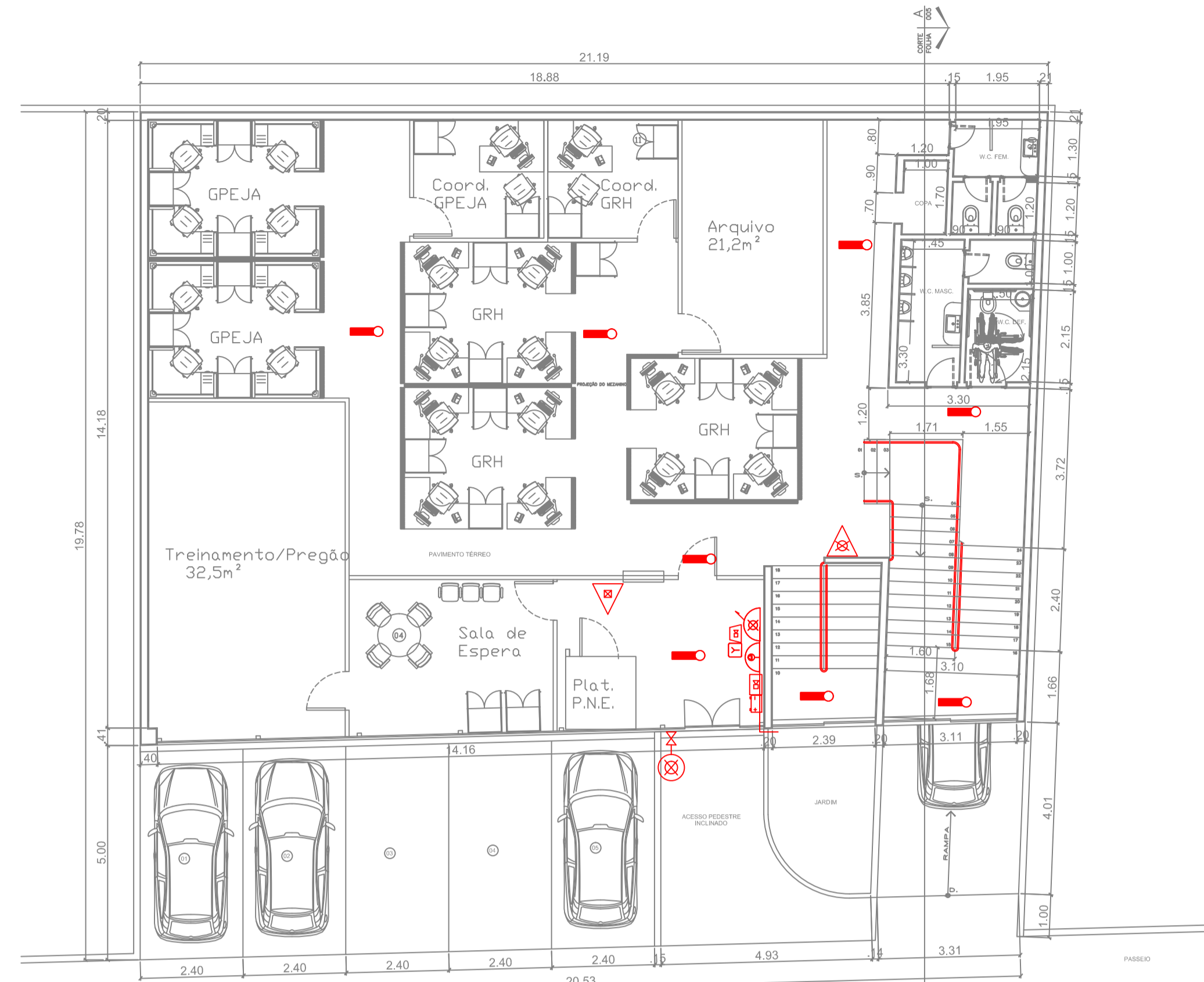
PLANTA BAIXA - PAVIMENTO TÉRREO Escala 1:100
